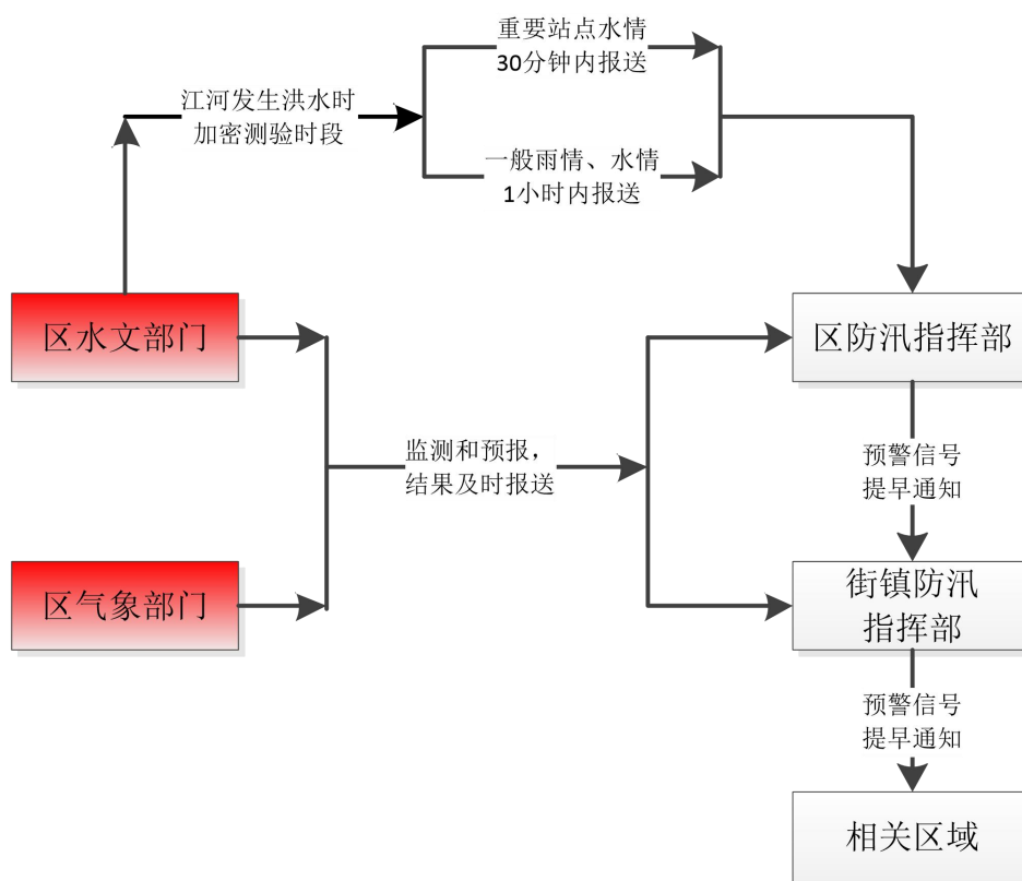
图2 气象水文信息预报预警流程图
