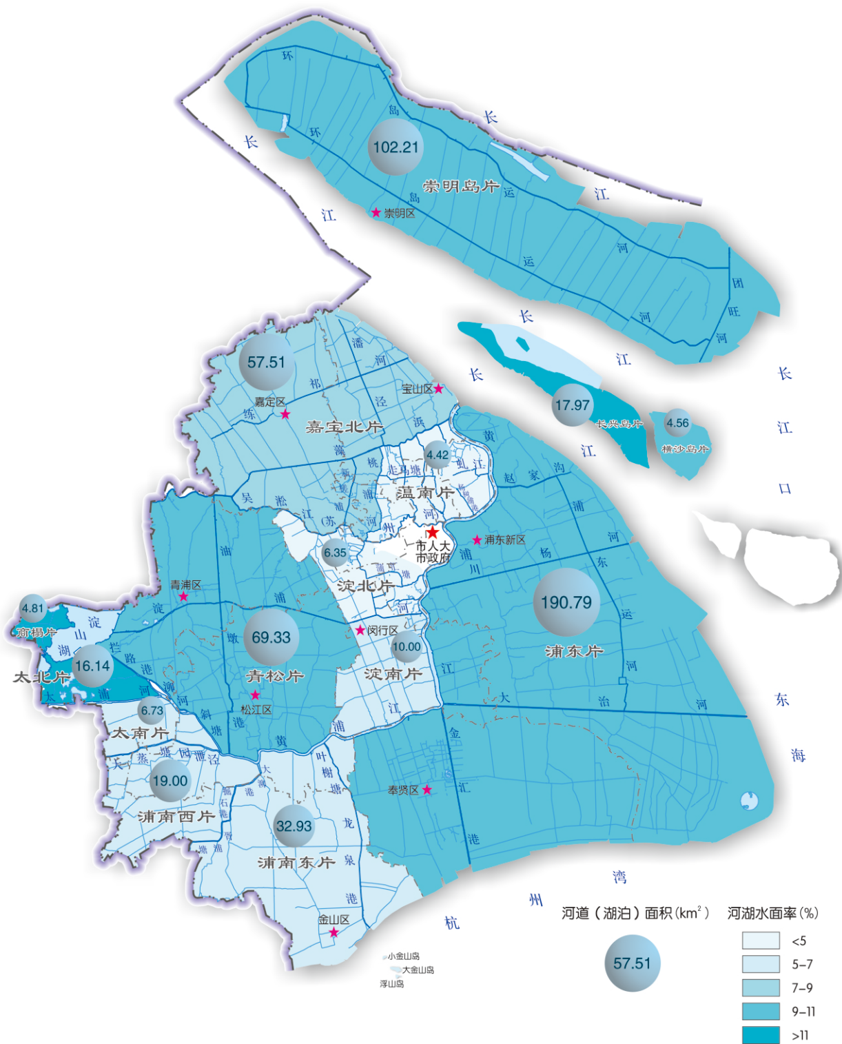
图3 2023年各水利片内河湖面积及河湖水面率统计图
