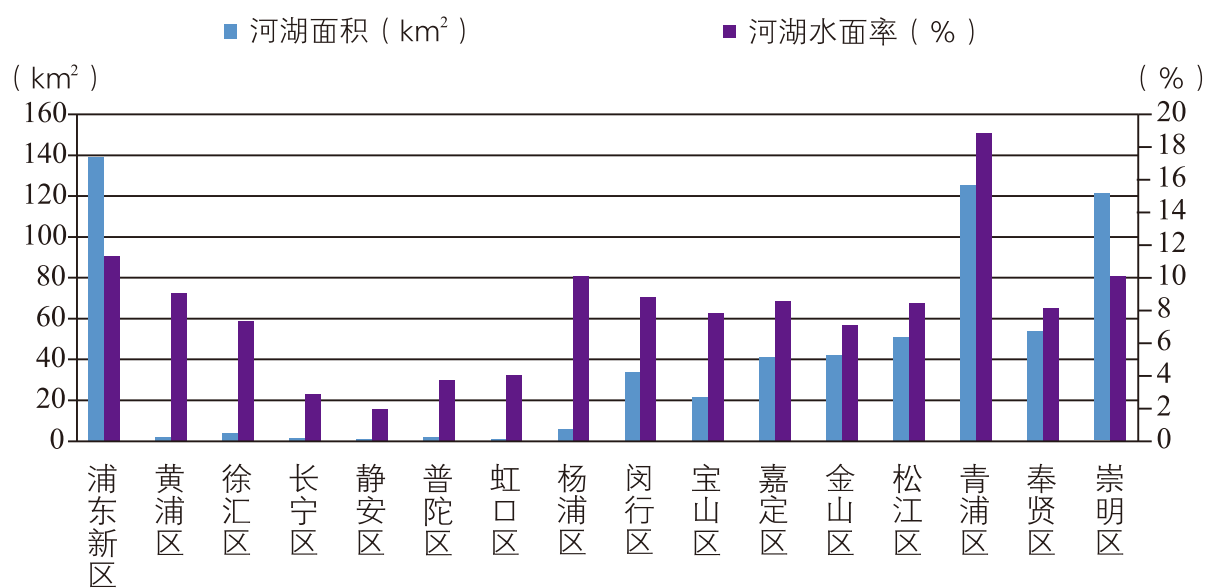
图4 2023年各区河湖面积、河湖水面率统计图
