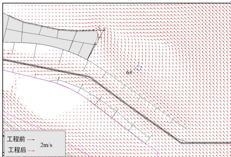
图 3.1-19 6#主采区采砂前后大潮涨急流场图（洪季）
