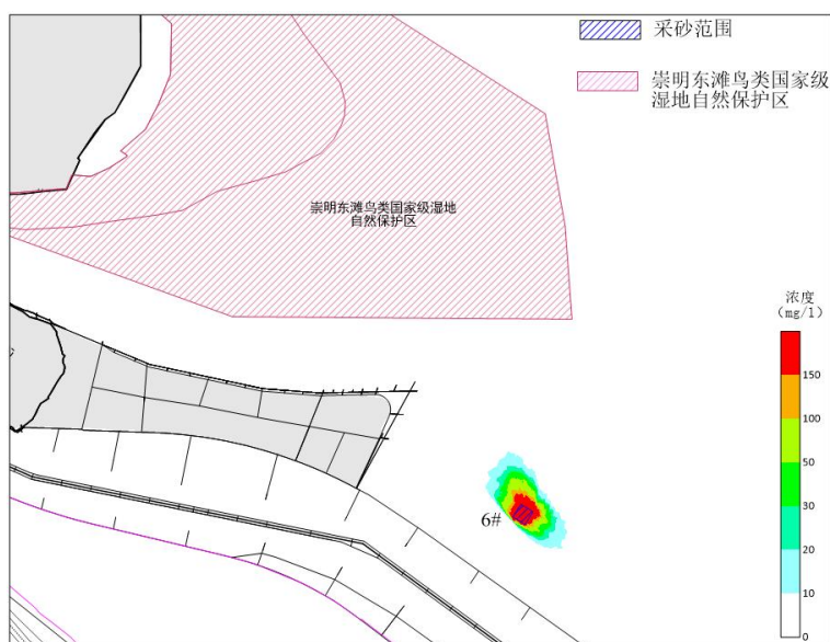
图 3.3-4 6#主采区施工悬浮物最大影响范围（枯季）
