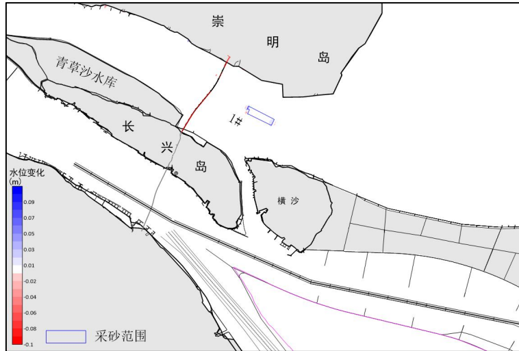
图 3.1-7 1#主采区采砂前后低水位变化图（洪季）
