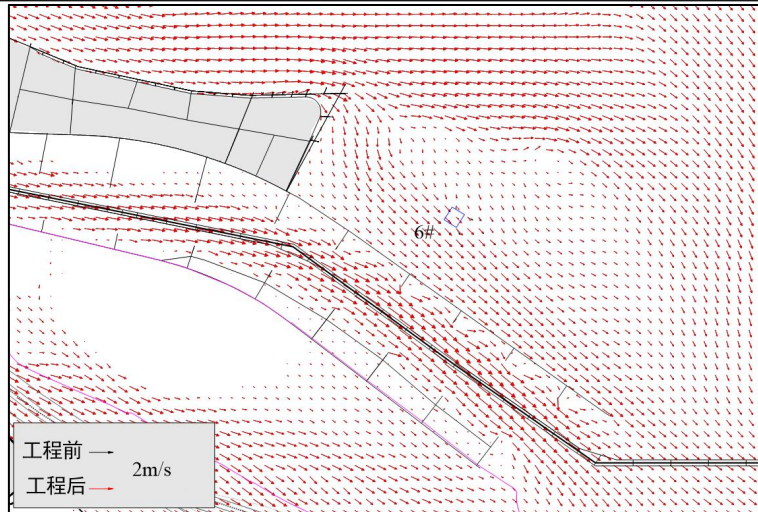
图 3.1-20 6#主采区采砂前后大潮落急流场图（洪季）
