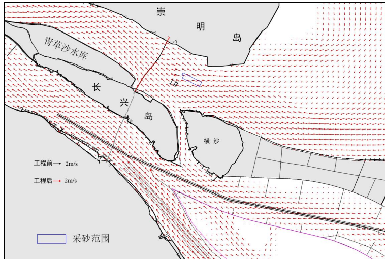
图 3.1-15 1#主采区采砂前后大潮涨急流场图（洪季）
