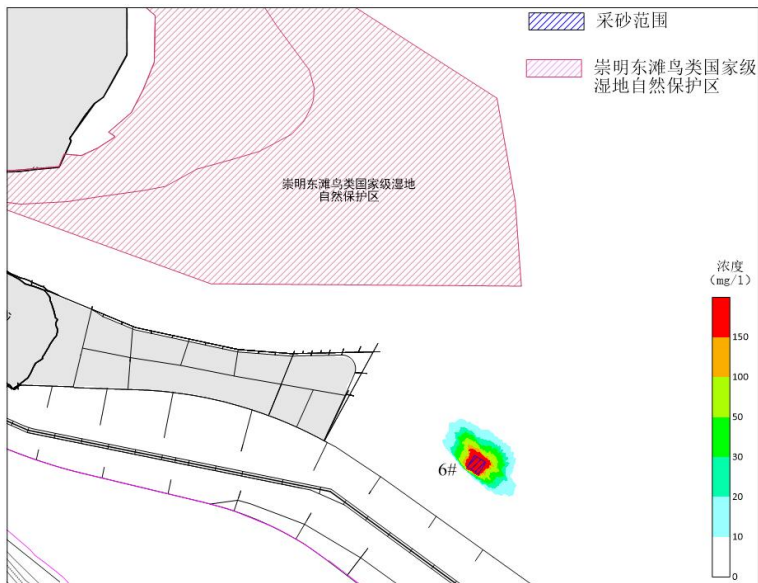
图 3.3-2 1#主采区施工悬浮物最大影响范围（枯季）
