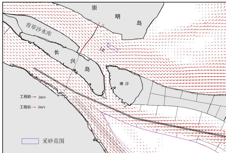
图 3.1-16 1#主采区采砂前后大潮落急流场图（洪季）
