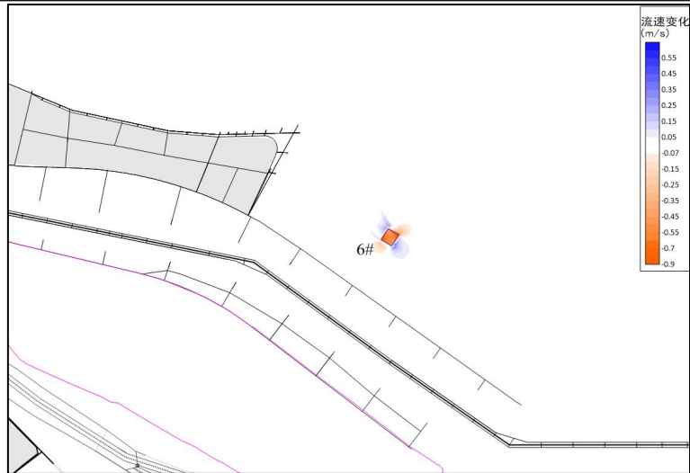
图 3.1-27 6#主采区采砂前后涨急流速差变化图（洪季）
