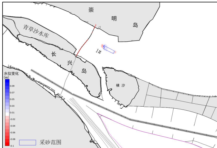
图 3.1-10 1#主采区采砂前后高水位变化图（枯季）
