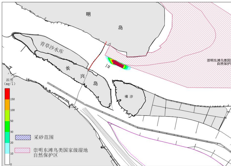
图 3.3-2 1#主采区施工悬浮物最大影响范围（枯季）
