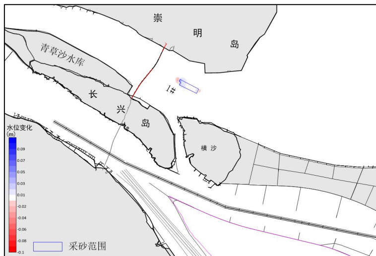
图 3.1-8 1#主采区采砂前后高水位变化图（洪季）
