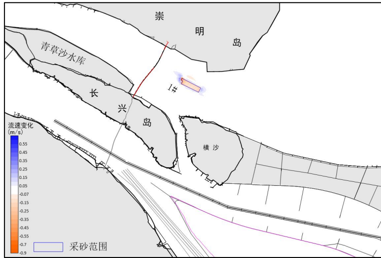
图 3.1-25 1#主采区采砂前后涨急流速差变化图（枯季）
