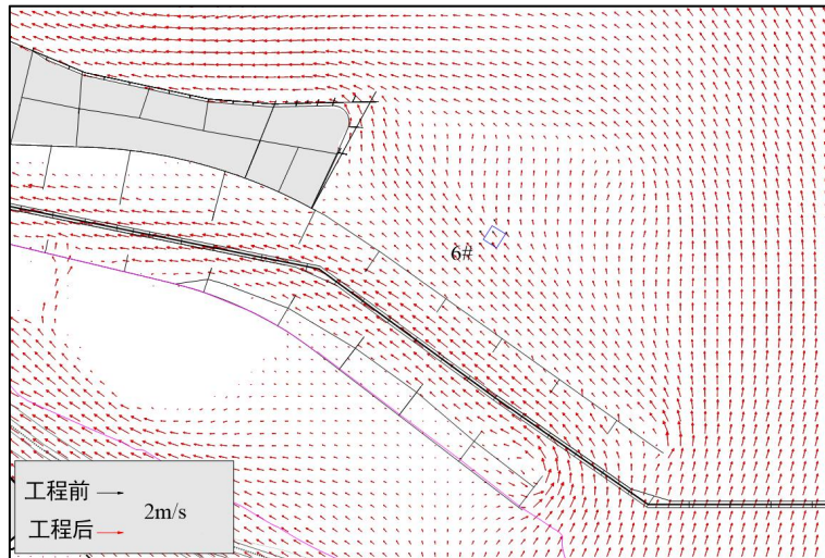
图 3.1-21 6#主采区采砂前后大潮涨急流场图（枯季）
