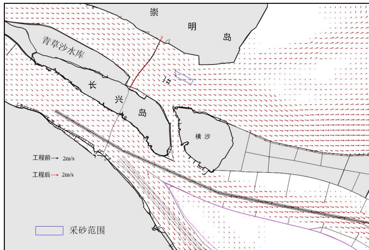
图 3.1-18 1#主采区采砂前后大潮落急流场图（枯季）
