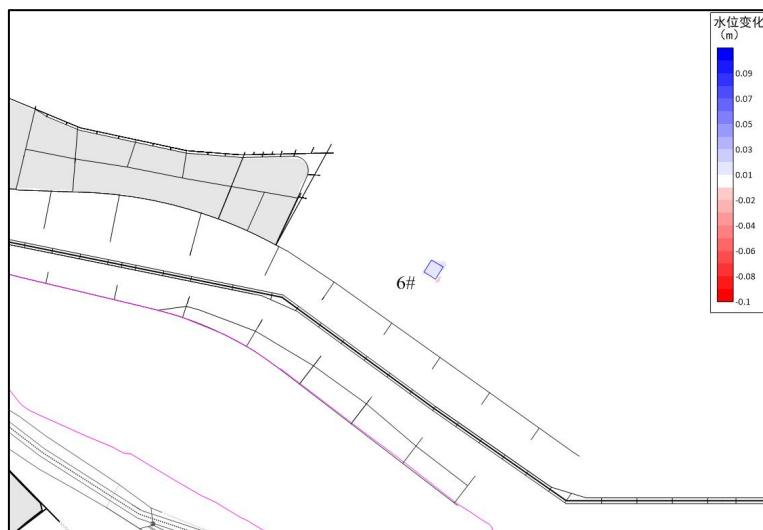
图 3.1-14 6#主采区采砂前后高水位变化图（枯季）
