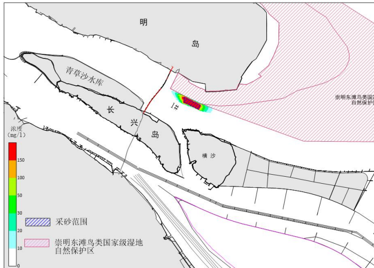
图 3.3-1 1#主采区施工悬浮物最大影响范围（洪季）
