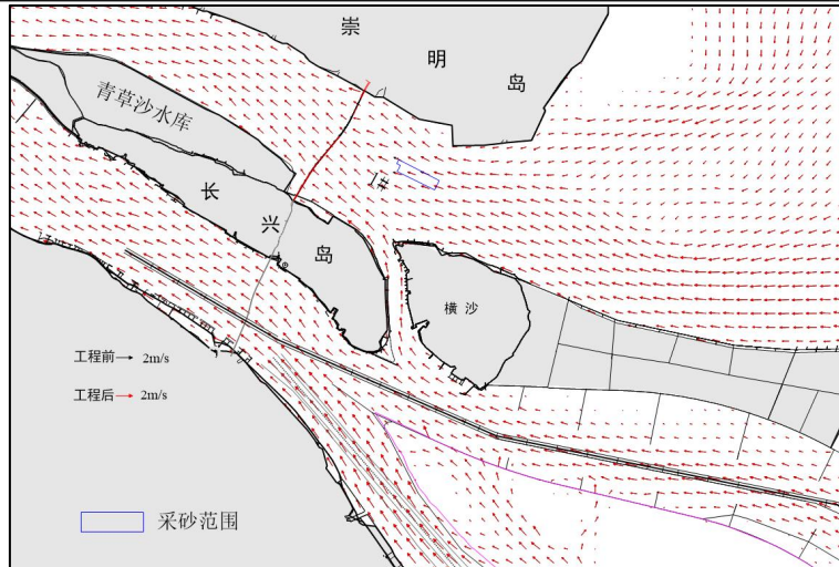
图 3.1-17 1#主采区采砂前后大潮涨急流场图（枯季）
