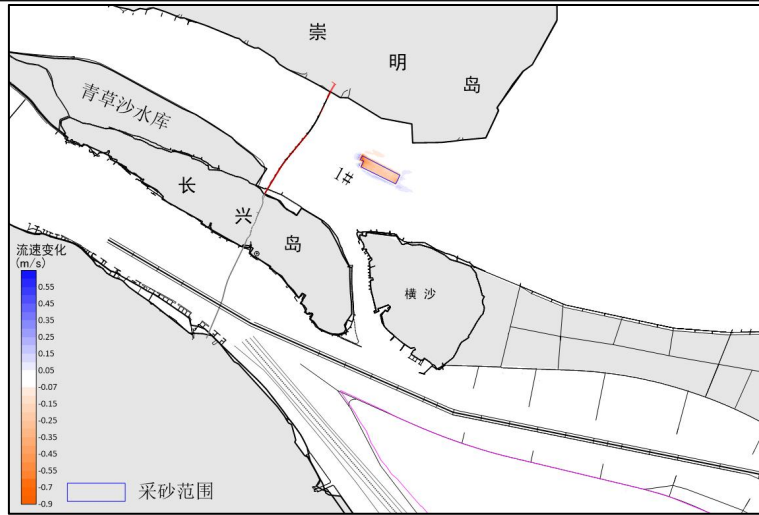
图 3.1-24 1#主采区采砂前后落急流速差变化图（洪季）
