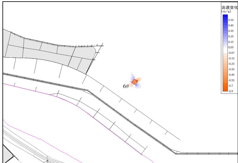
图 3.1-28 6#主采区采砂前后落急流速差变化图（洪季）
