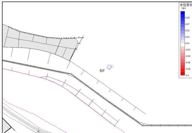
图 3.1-13 6#主采区采砂前后低水位变化图（枯季）
