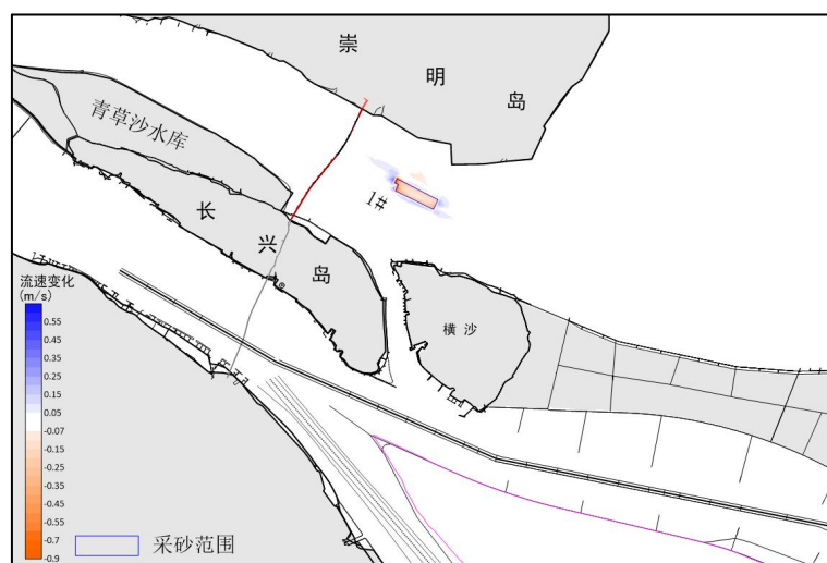
图 3.1-23 1#主采区采砂前后涨急流速差变化图（洪季）
