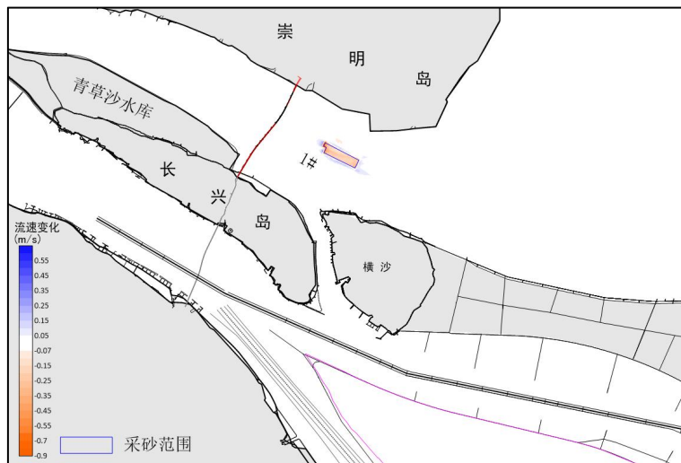
图 3.1-26 1#主采区采砂前后落急流速差变化图（枯季）
