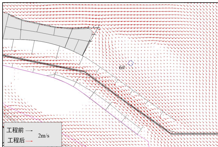
图 3.1-22 6#主采区采砂前后大潮落急流场图（枯季）
