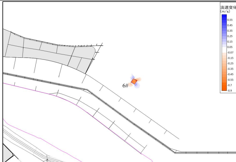
图 3.1-30 6#主采区采砂前后落急流速差变化图（枯季）
