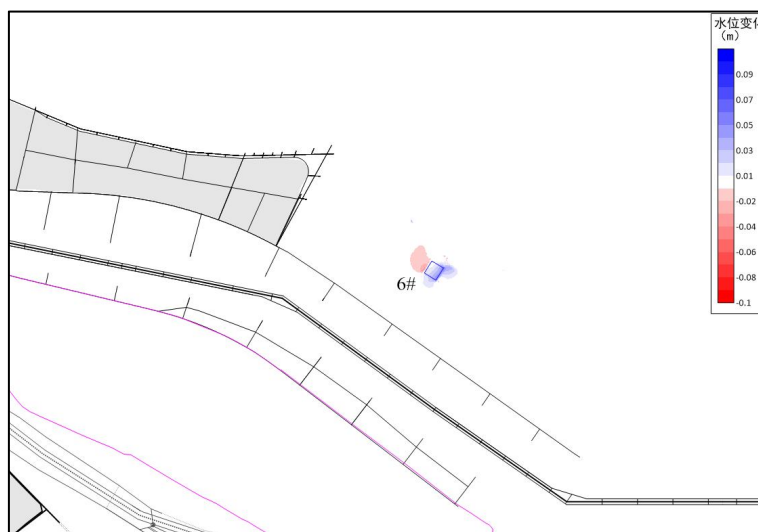
图 3.1-11 6#主采区采砂前后低水位变化图（洪季）
